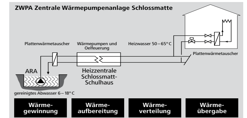
Von der Wärmegewinnung in der ARA Münsingen bis zur Wärmeübergabe in der angeschlossenen Liegenschaft
